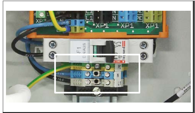
Abb. 1: Beispiel für einen Netzanschluss
